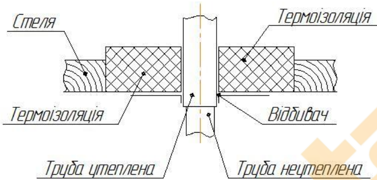
Малюнок 6. Проходження димоходу крізь стелю
