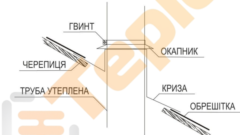
Малюнок 7. Проходження димоходу крізь кришу
